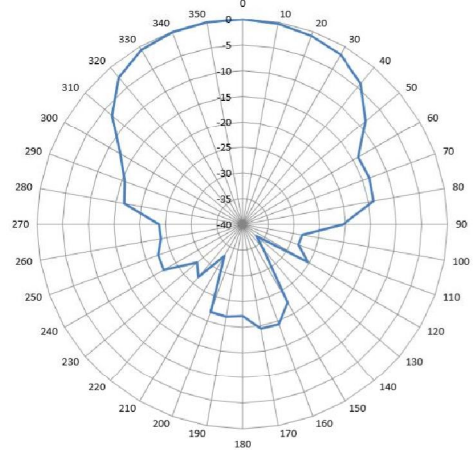
4.7GHz ビームパターン (44Sa53M)
