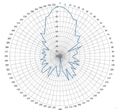
28GHz ビームパターン (44Sa53H)
