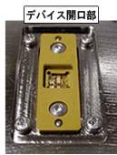
自動嵌合治具 (エア使用)
