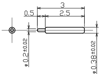
プローブピン 参考図
