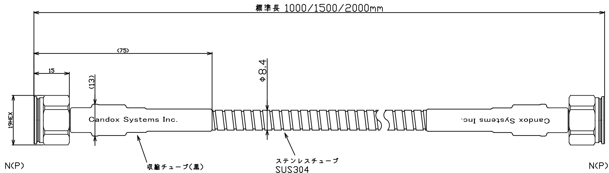
ケーブル構造 (mm)
