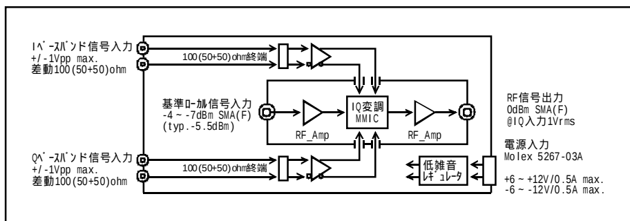
構成図
