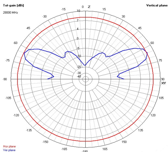
2D水平垂直放射パターンイメージ
