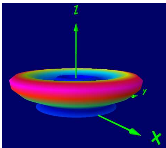
3D放射パターンイメージ
